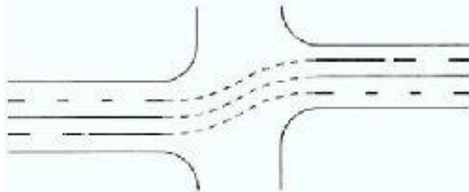
Marcaj de ghidare la traversarea unei intersecții
